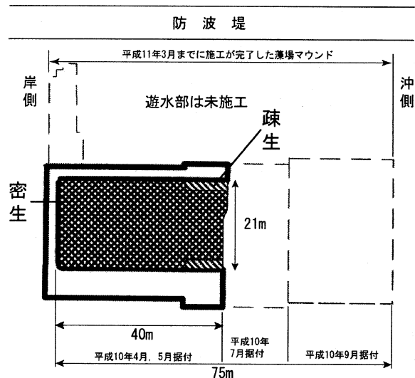
図-3 平成11年3月の藻場分布
